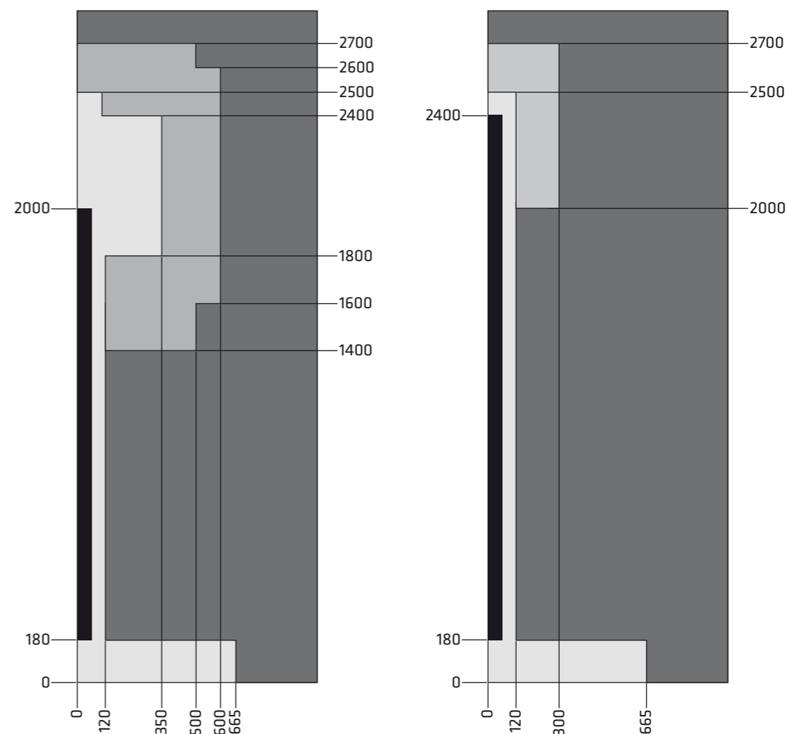
Veiligheidsafstanden volgens DIN EN ISO 13857
