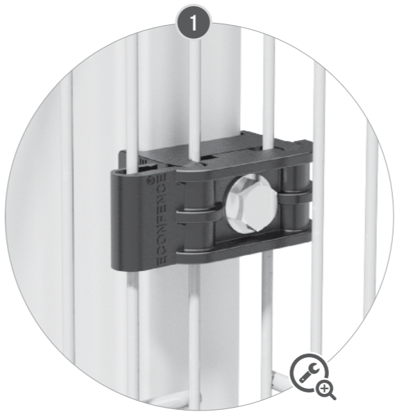
Ansicht voltooide Montage van de klemelementen ZB31004
